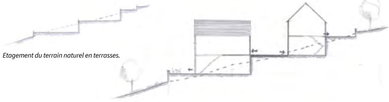
Implantation des maisons en profitant du dénivelé, gestion d'accès haut et bas.
